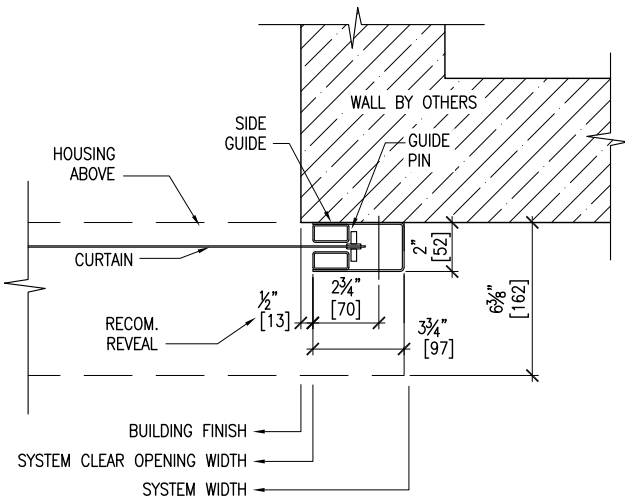
(D) GUIDE DETAIL 1 1/2" = 1'-0"
