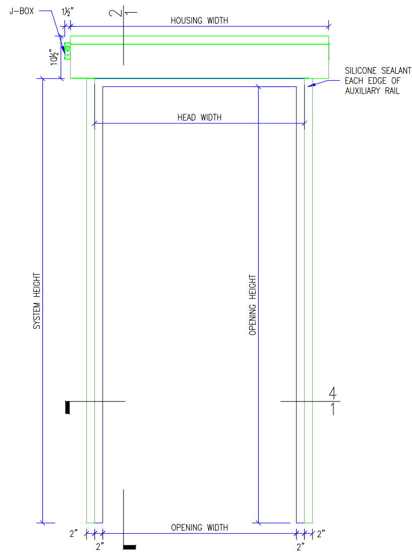
① M200 ELEVATION SCALE: 1/2" = 1'-0"
